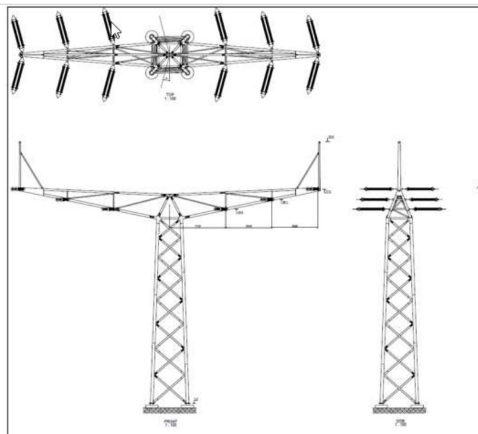
Figur 4 Afspændingsknækmast
